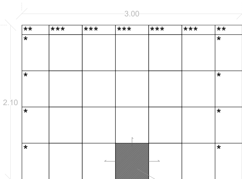
DESPIECES MURO G DALTILE NIRVANA BLACK RECTIFICADO
