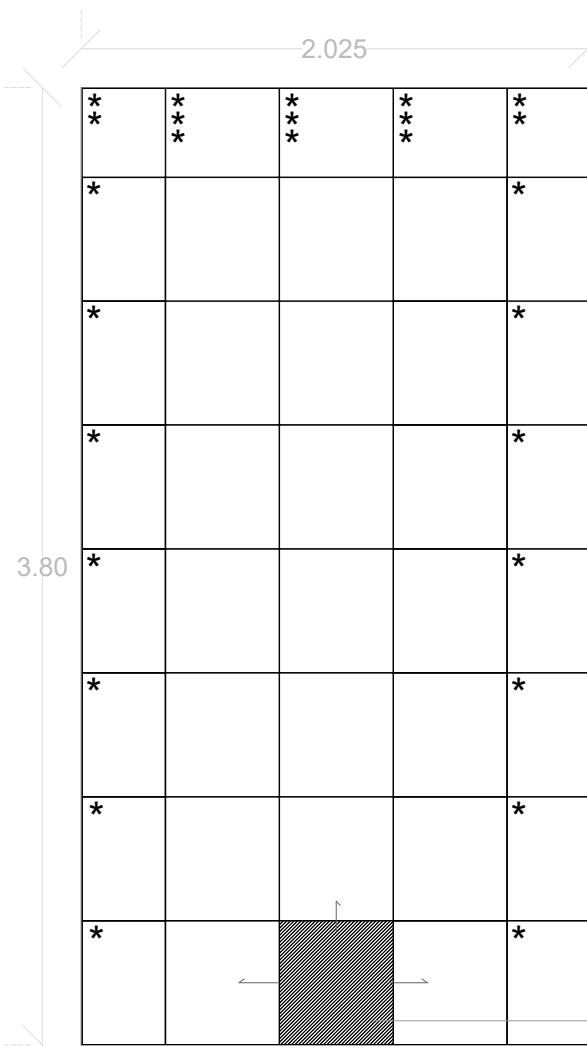
DESPIECES MURO D DALTILE NIRVANA BLACK RECTIFICADO
