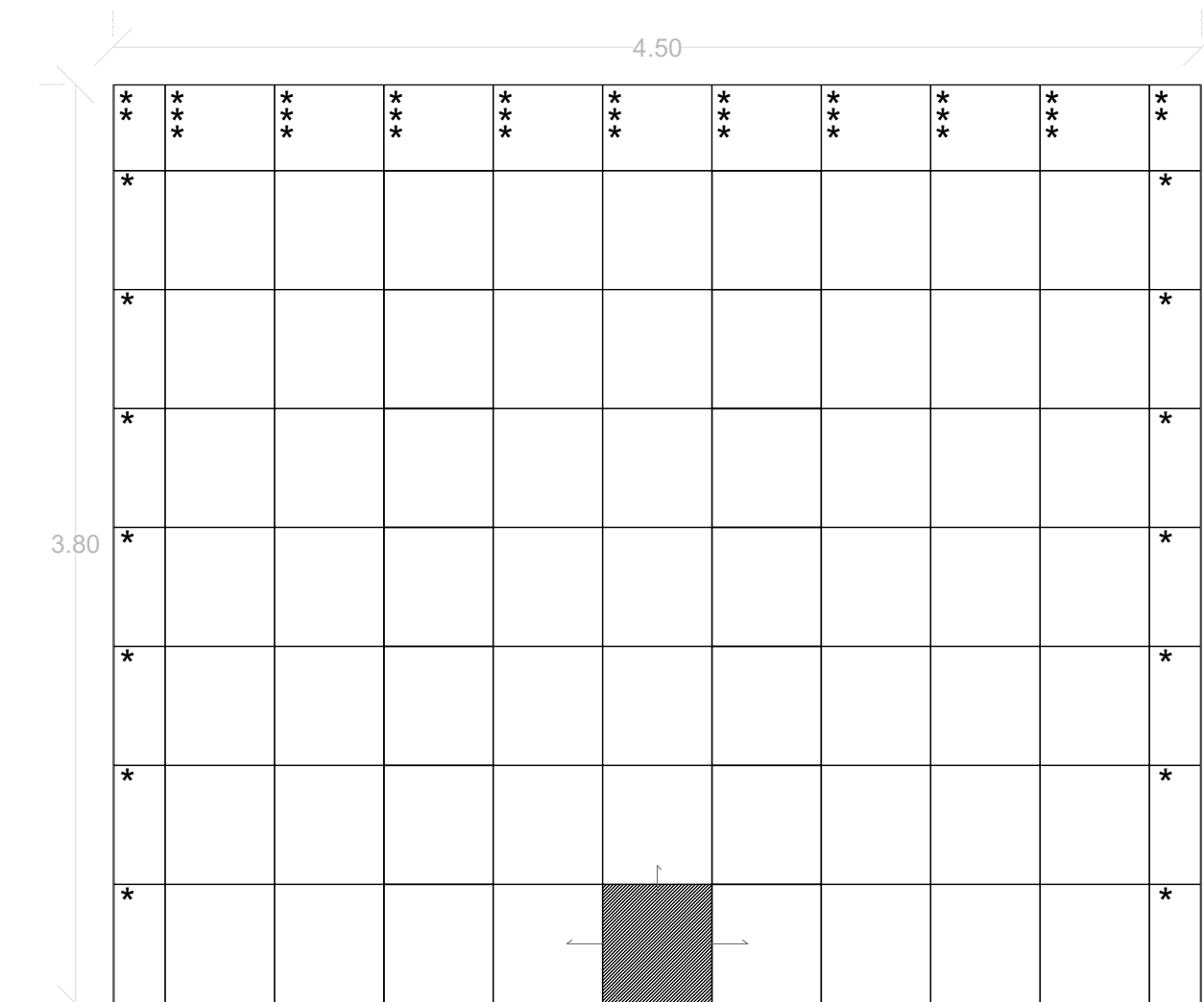
DESPIECES MURO F DALTILE NIRVANA BLACK RECTIFICADO
