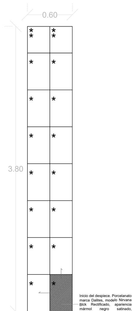
DESPIECES MURO H DALTILE NIRVANA BLACK RECTIFICADO
