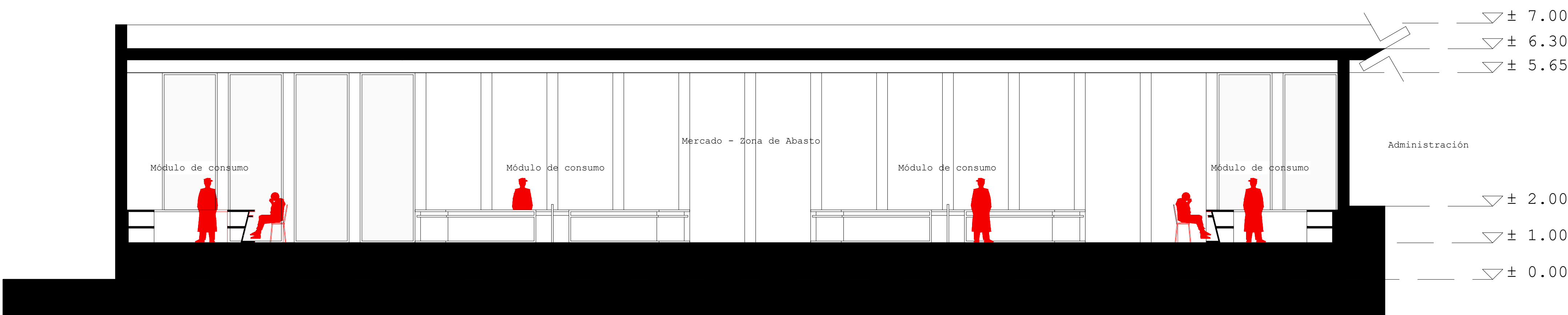
CORTE LONGITUDINAL 1
