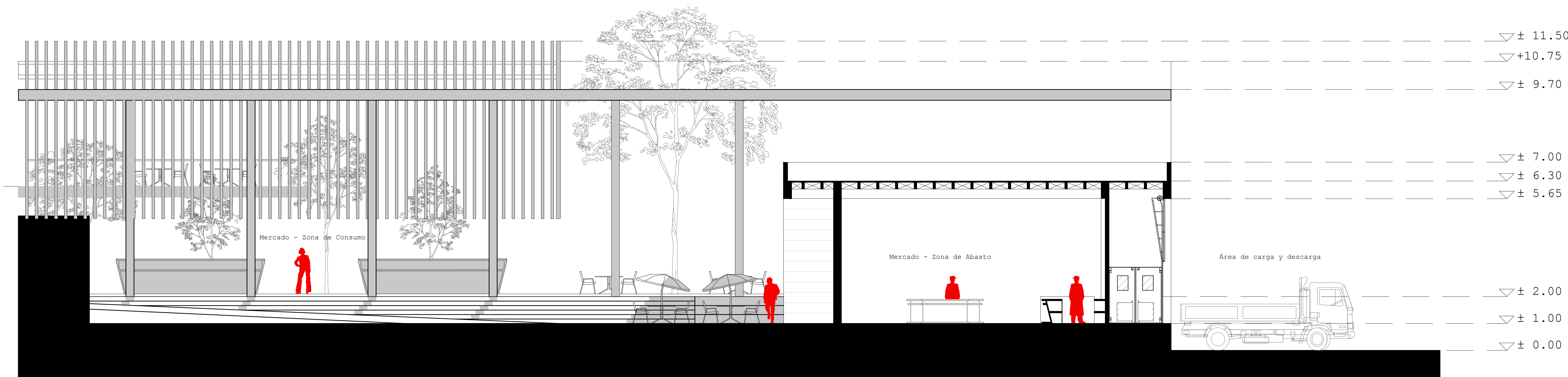
CORTE TRANSVERSAL 1
