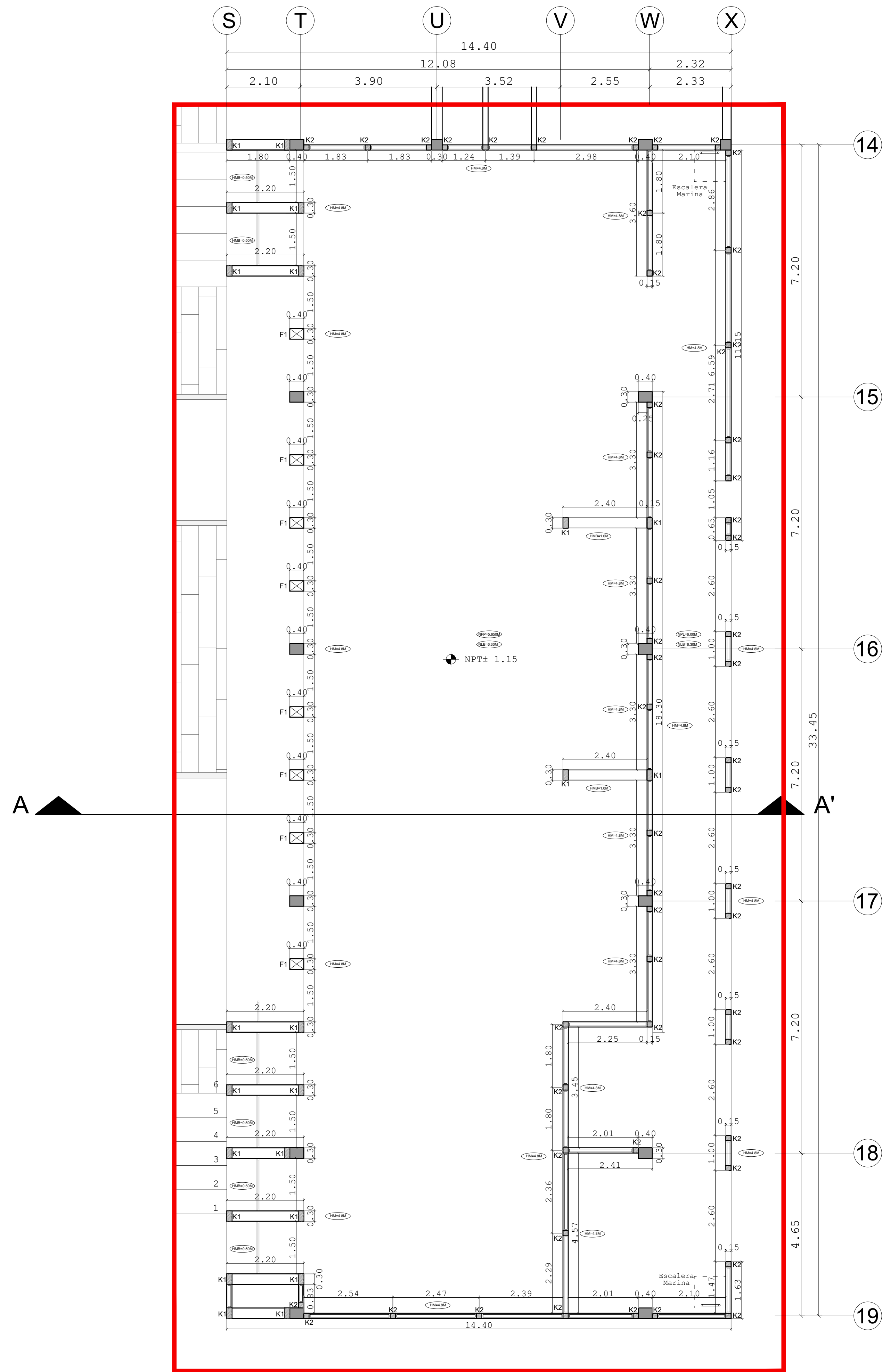
PLANTA SECCIÓN 1
