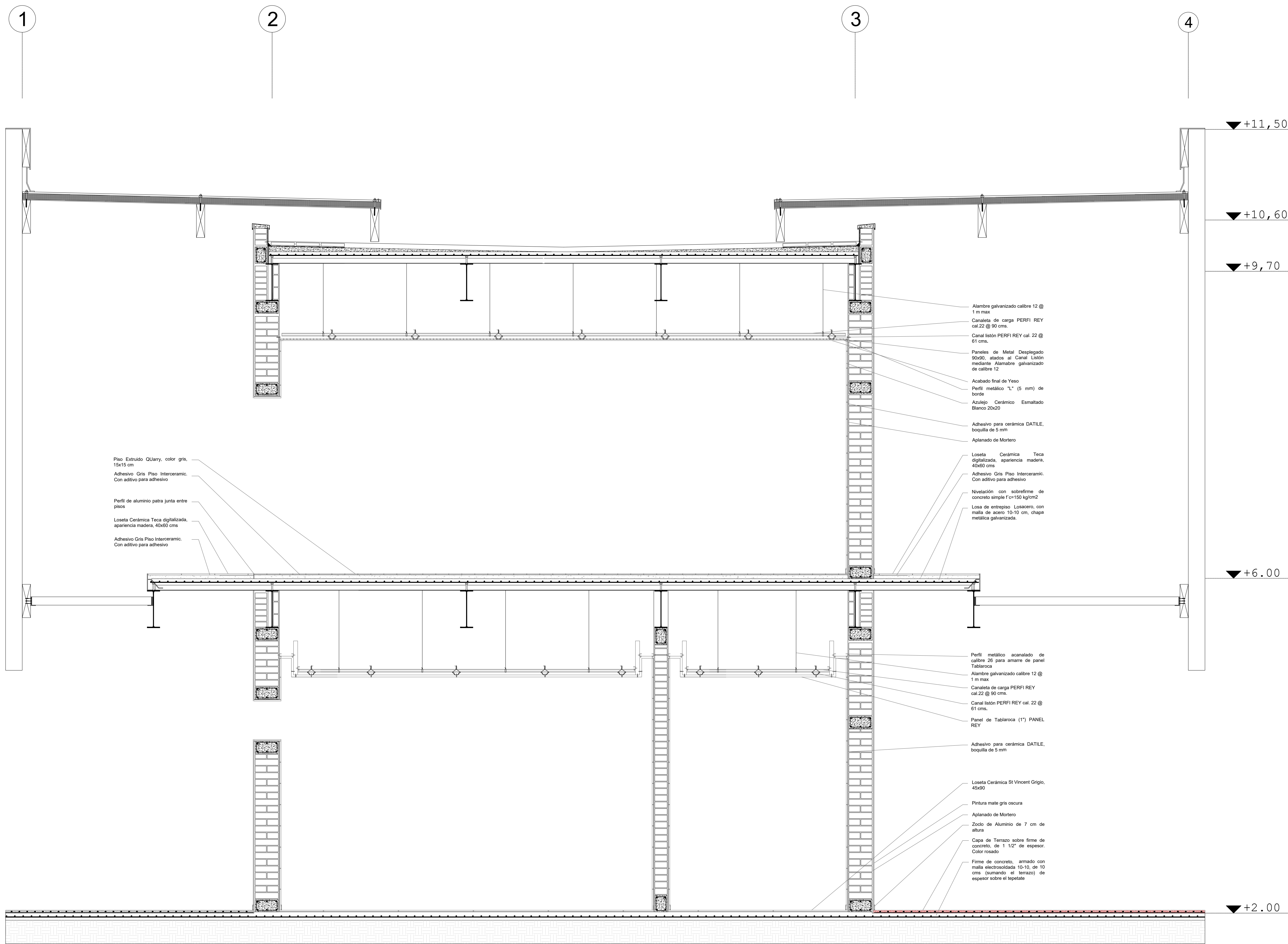
CORTE POR FACHADA VOL. RESTAURANTES
