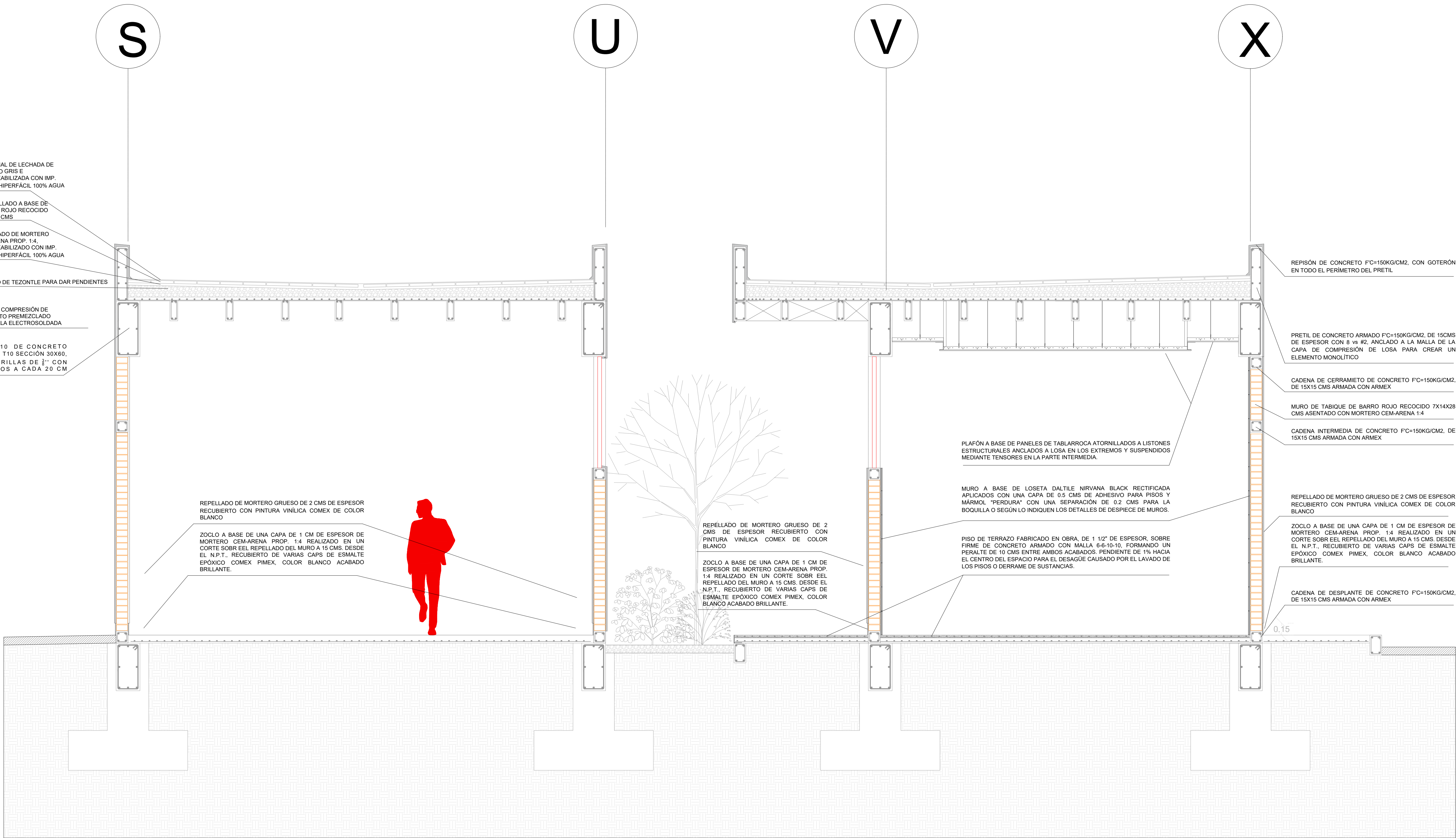
CORTE POR FACHADA ZONA DE SERVICIOS DEL MERCADO
